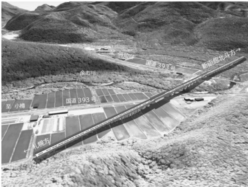
明治高架橋工区の完成予想図 (国土地理院基盤地図情報及び地理院タイルを加工して作成)
