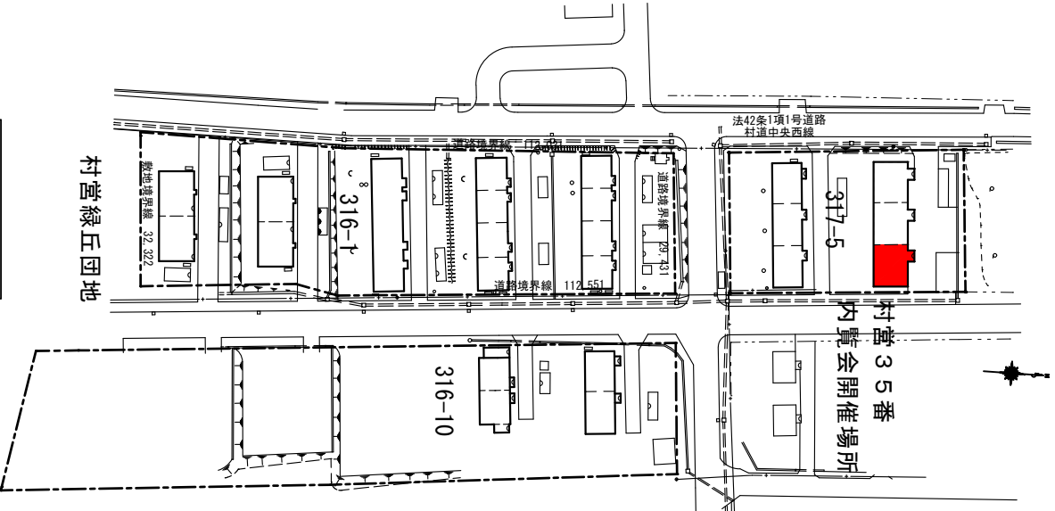
団地配置図 S: 1/500
